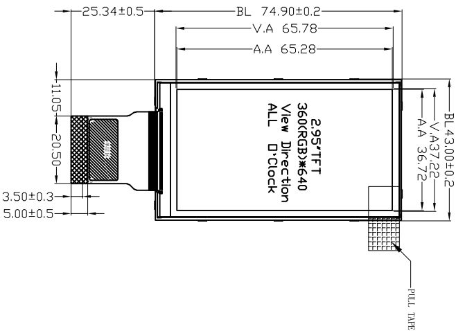
正视图
