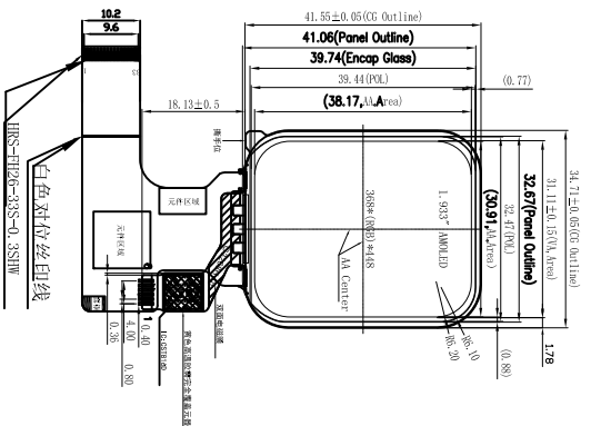
正视图
