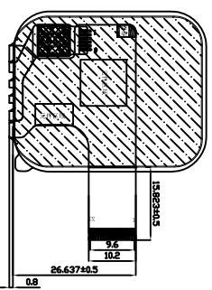
弯折示意图 弯折固定出货
