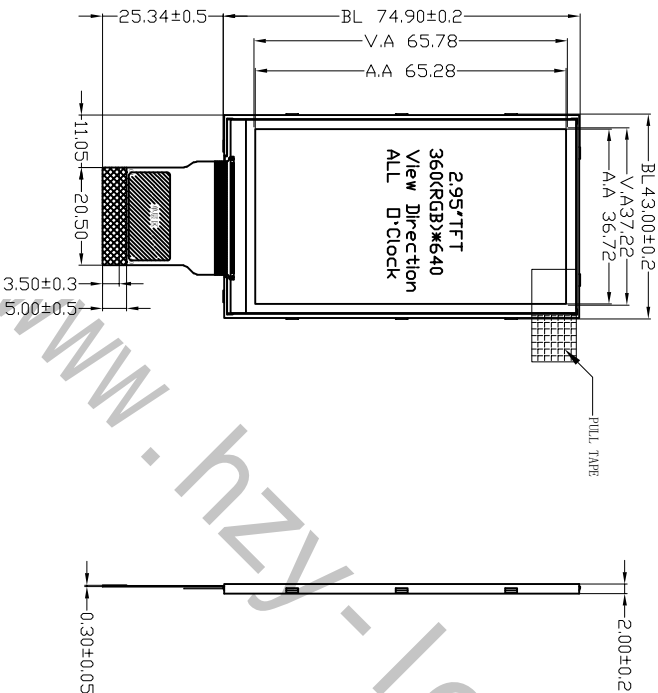
正视图
