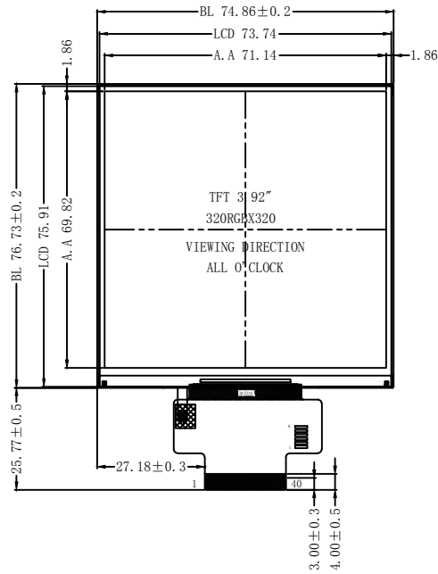
正视图
